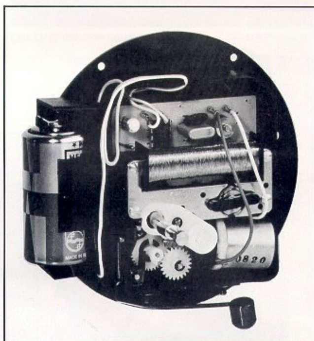
Schiffsquarzwerk mit Glasenschlag
