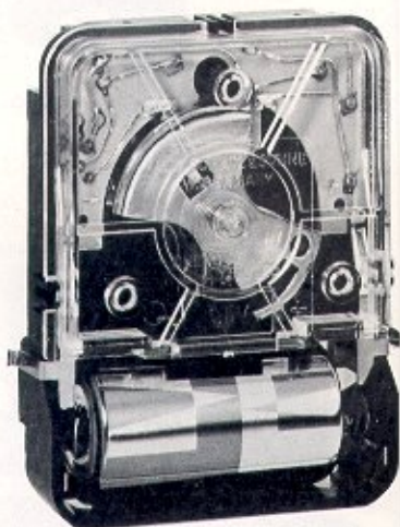
Pendelaggregat der heutigen Quarz-Jahresuhr
