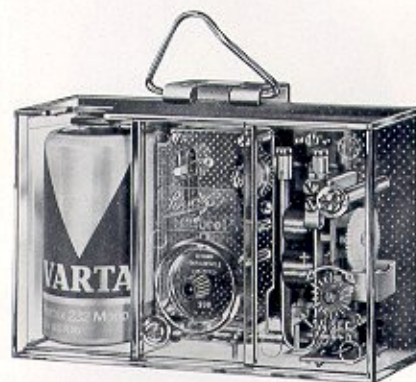
1970 Stimmgabelwerk
